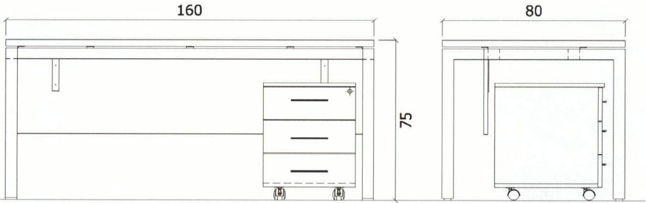
ÖN GÖRÜNÜS
