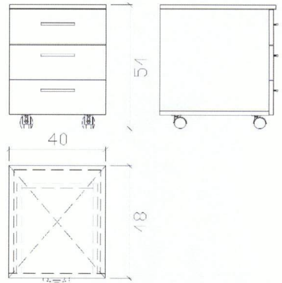
YAN GÖRÜNÜS
